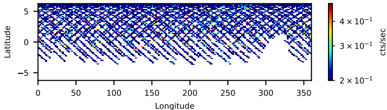
60701013002: 3 to 10 keV
