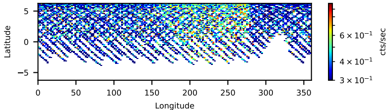
60701013002: 30 to 120 keV
