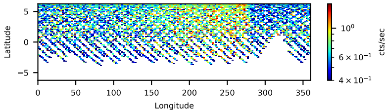
60701013002: 3 to 120 keV
