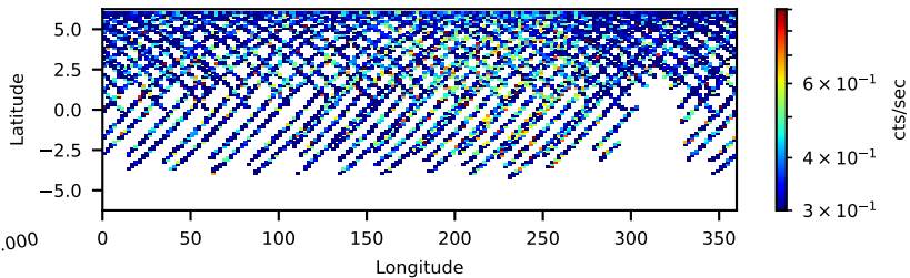
60668003002: 30 to 120 keV
