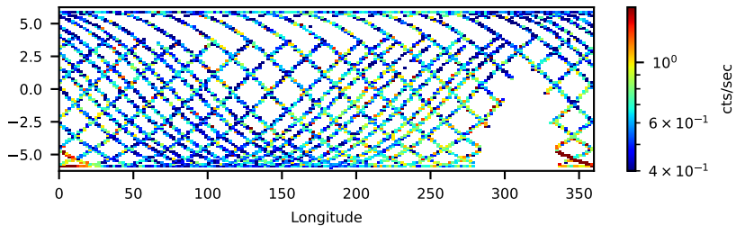
60666012002: 3 to 10 keV
