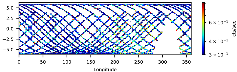
60666012002: 30 to 120 keV
