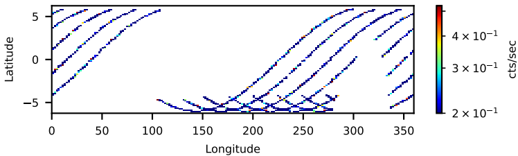
60662001006: 3 to 10 keV
