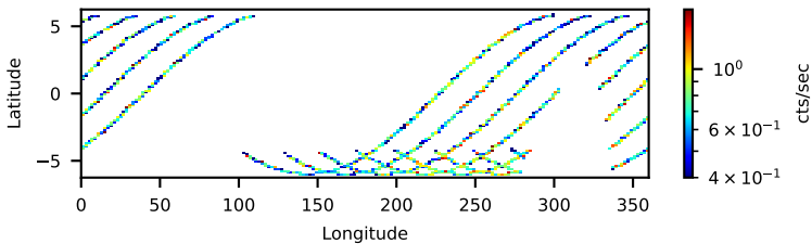
60662001006: 3 to 120 keV
