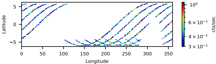
60662001006: 30 to 120 keV
