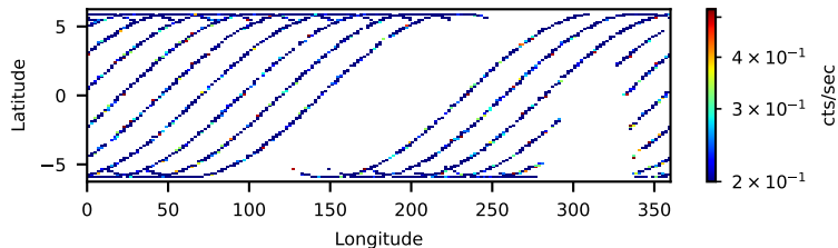
60602003002: 3 to 10 keV
