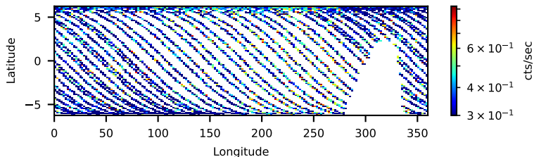
60601028002: 30 to 120 keV
