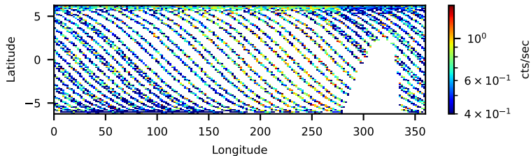
60601028002: 3 to 120 keV
