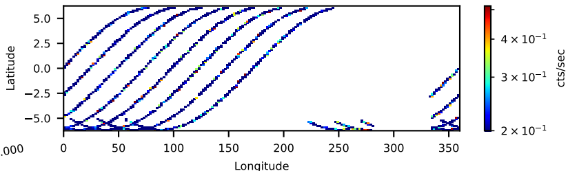
60502053002: 30 to 120 keV
