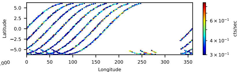
60502053002: 30 to 120 keV
