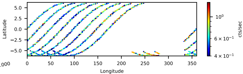
60502053002: 3 to 10 keV
