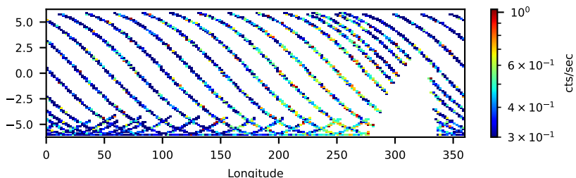
60502006004: 30 to 120 keV
