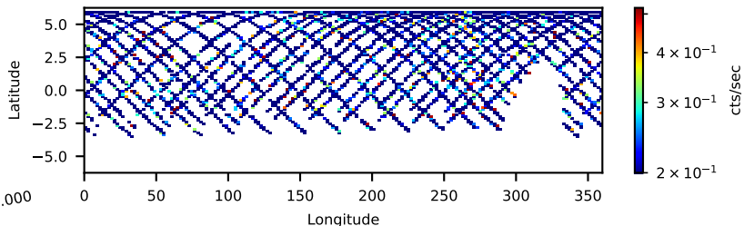
60501031004: 30 to 120 keV
