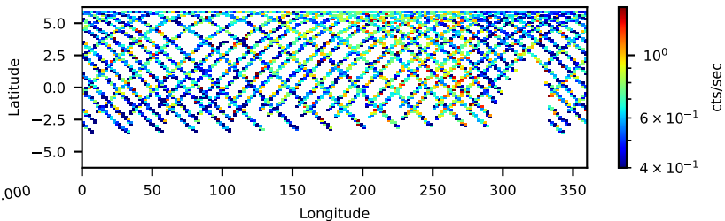
60501031004: 3 to 10 keV
