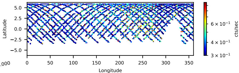
60501031004: 30 to 120 keV
