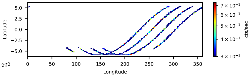
60464083002: 30 to 120 keV
