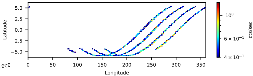
60464083002: 3 to 10 keV
