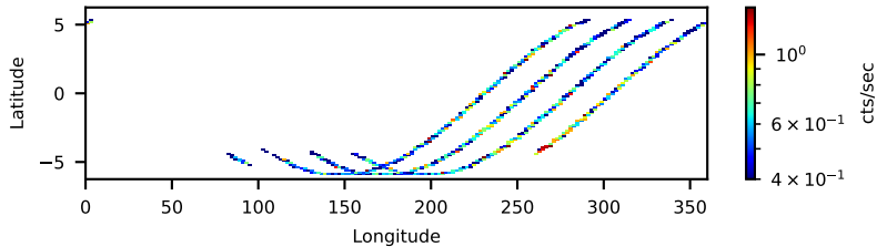
60464083002: 3 to 120 keV
