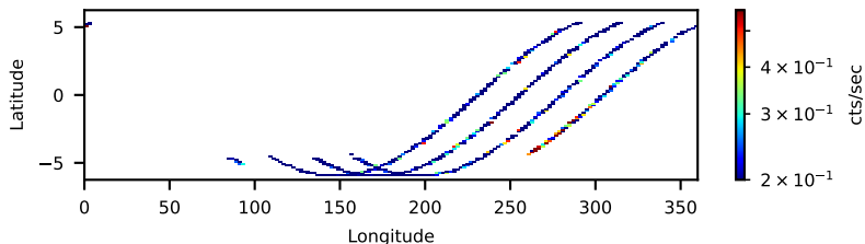
60464083002: 3 to 10 keV
