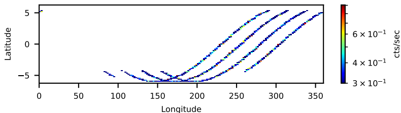
60464083002: 30 to 120 keV
