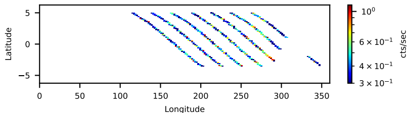
60464014002: 30 to 120 keV
