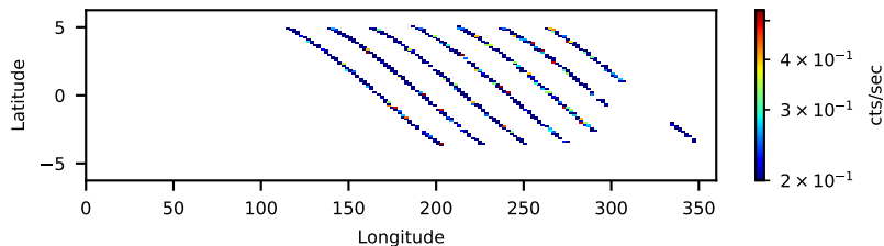
60464014002: 3 to 10 keV
