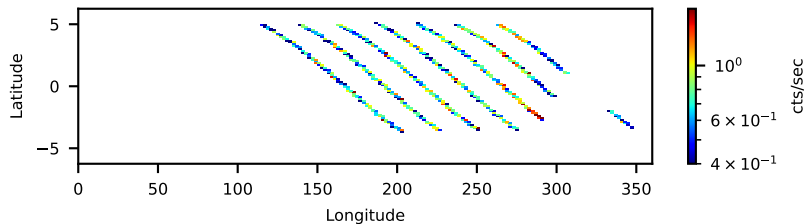
60464014002: 3 to 120 keV
