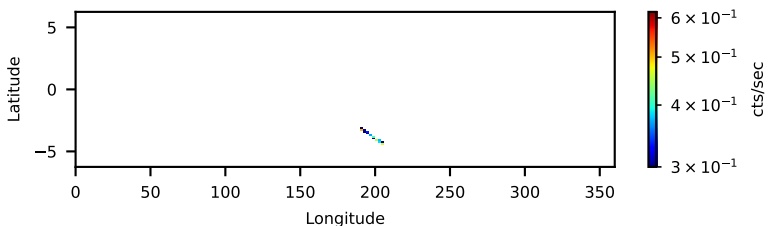
60464005001: 30 to 120 keV
