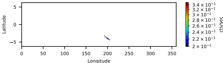
60464005001: 3 to 10 keV
