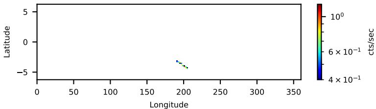
60464005001: 3 to 120 keV
