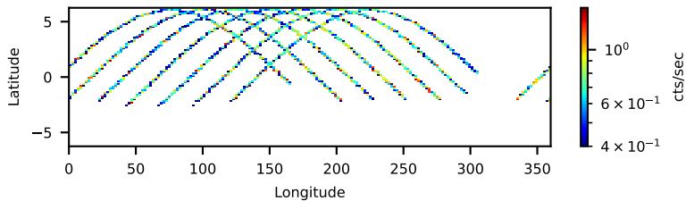
60463013002: 3 to 120 keV
