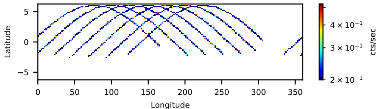
60463013002: 3 to 10 keV
