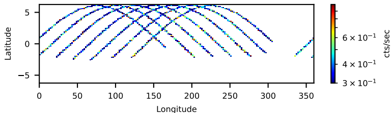
60463013002: 30 to 120 keV
