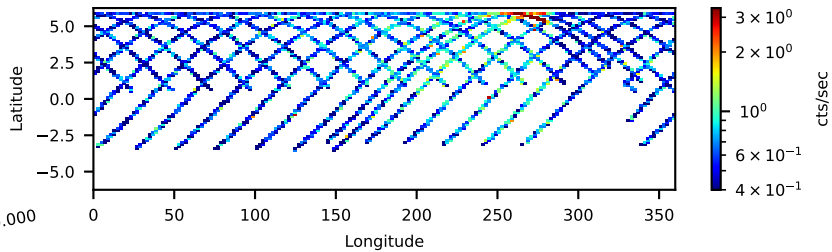
60402021008: 3 to 10 keV
