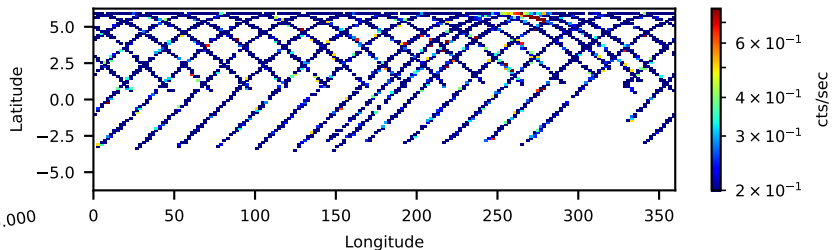
60402021008: 30 to 120 keV
