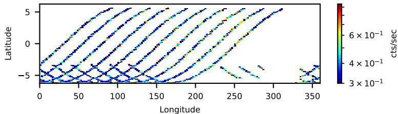
60402003004: 30 to 120 keV
