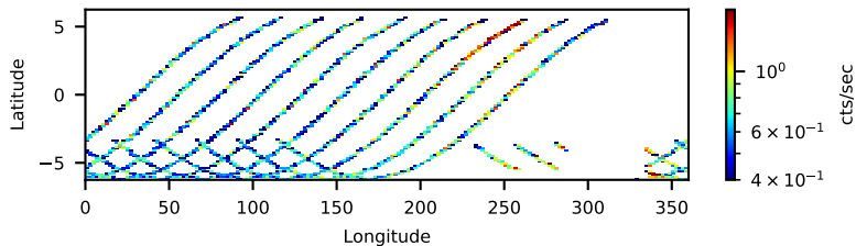
60402003004: 3 to 120 keV
