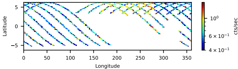
60376005002: 3 to 120 keV
