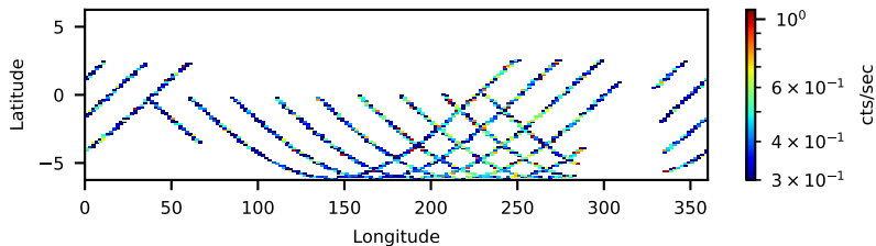
60374003002: 30 to 120 keV
