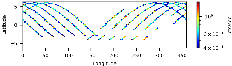
60374001002: 3 to 120 keV
