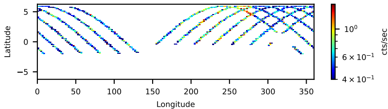
60367001002: 3 to 120 keV
