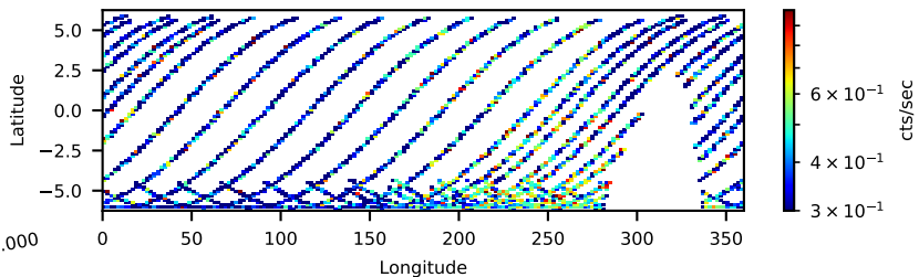
60364002002: 30 to 120 keV
