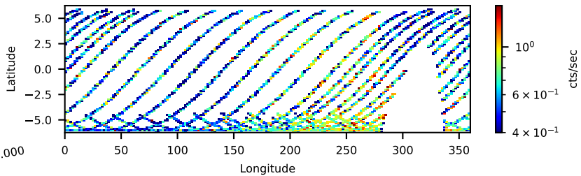
60364002002: 3 to 10 keV
