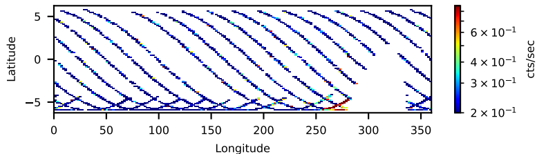
60362026002: 3 to 10 keV
