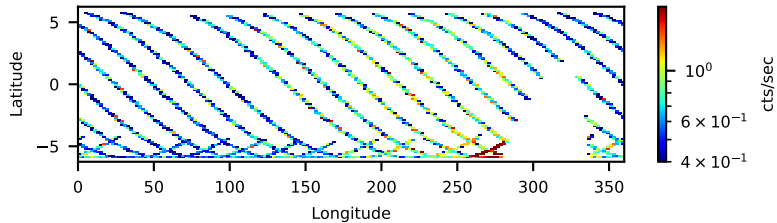
60362026002: 3 to 120 keV
