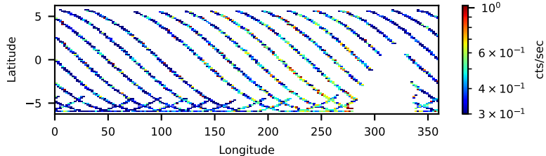
60362026002: 30 to 120 keV
