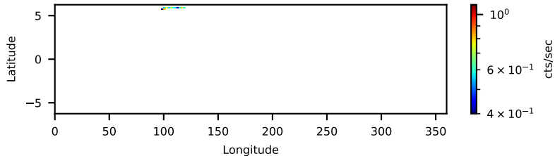
60301029001: 3 to 120 keV
