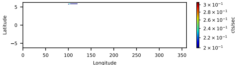
60301029001: 3 to 10 keV
