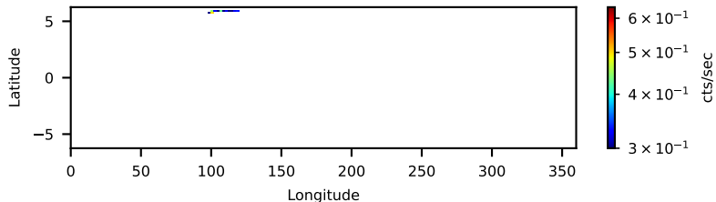
60301029001: 30 to 120 keV
