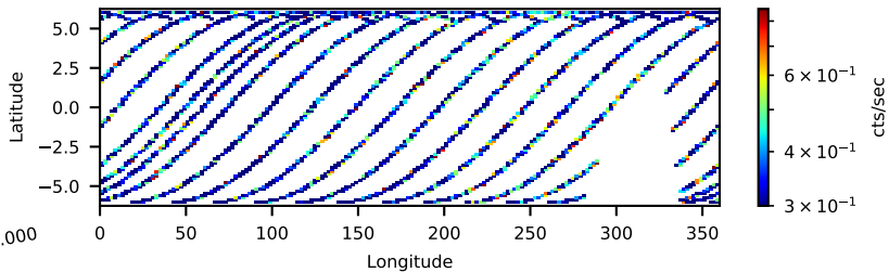
60301027002: 30 to 120 keV
