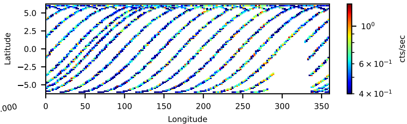
60301027002: 3 to 10 keV
