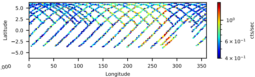
60301026002: 3 to 10 keV
