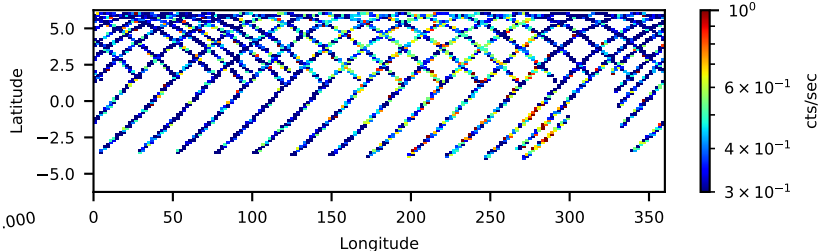
60301026002: 30 to 120 keV
