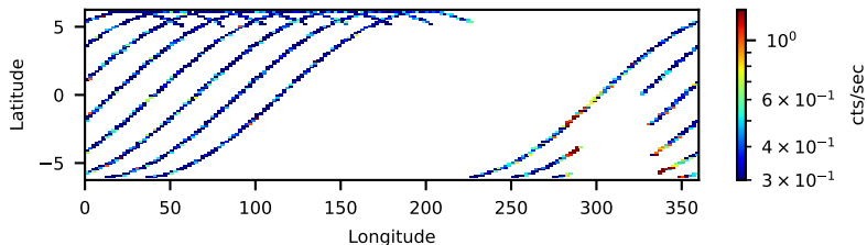
60260006002: 30 to 120 keV
