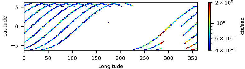
60260006002: 3 to 120 keV
