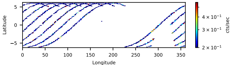
60260006002: 3 to 10 keV
