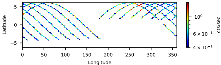
60202015004: 3 to 120 keV
