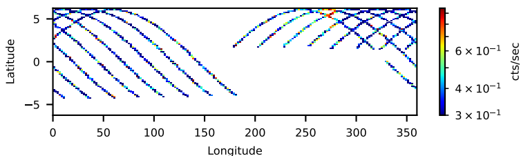
60202015004: 30 to 120 keV
