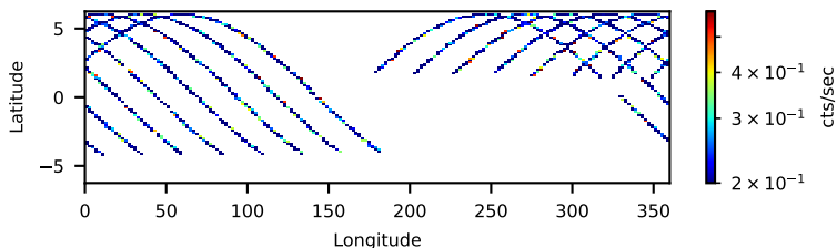
60202015004: 3 to 10 keV
