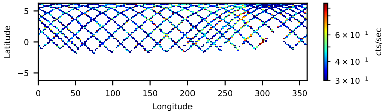
60201063002: 30 to 120 keV
