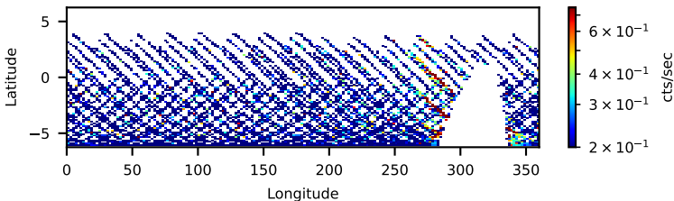
60201057002: 3 to 10 keV
