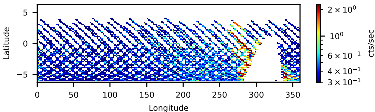
60201057002: 30 to 120 keV
