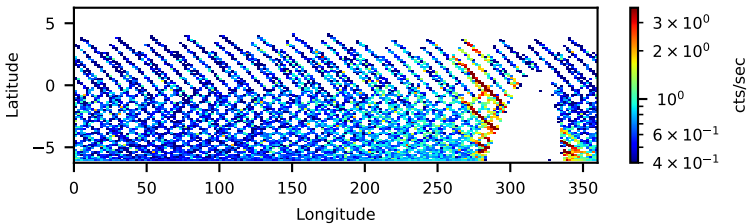
60201057002: 3 to 120 keV
