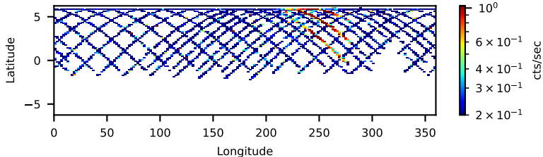
60201056002: 3 to 10 keV
