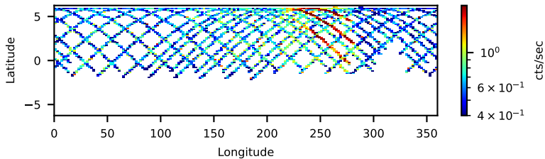
60201056002: 3 to 120 keV
