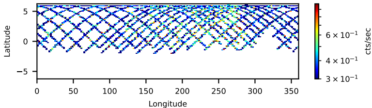
60201056002: 30 to 120 keV
