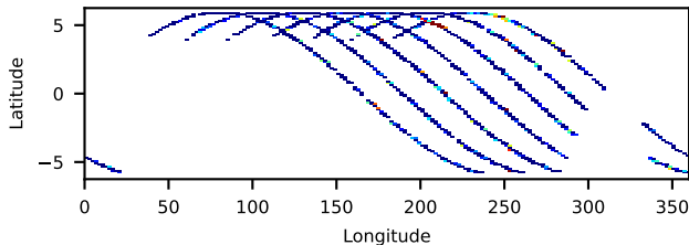
60161123002: 3 to 10 keV
