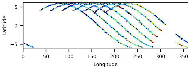
60161123002: 3 to 120 keV
