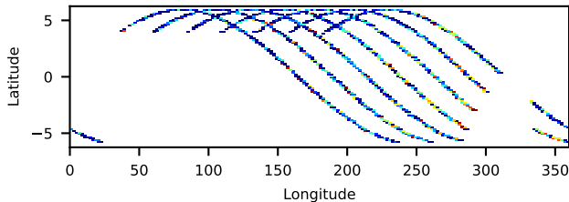
60161123002: 30 to 120 keV
