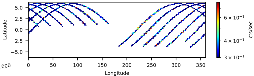
60161025002: 30 to 120 keV
