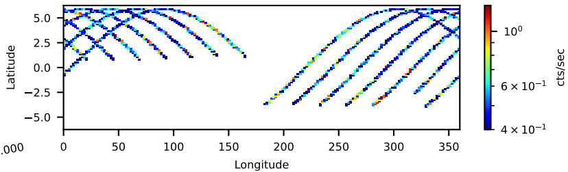
60161025002: 3 to 10 keV
