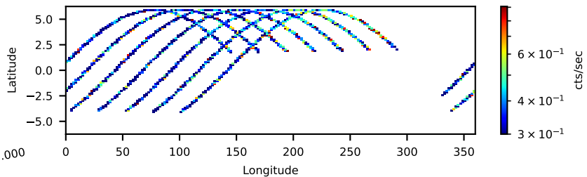
60160768002: 30 to 120 keV
