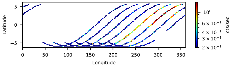
60160745002: 3 to 10 keV
