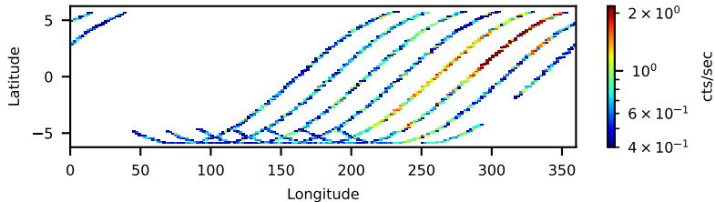
60160745002: 3 to 120 keV
