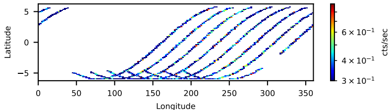
60160745002: 30 to 120 keV
