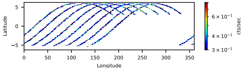
60160663002: 30 to 120 keV
