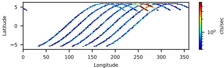
60160625002: 3 to 120 keV
