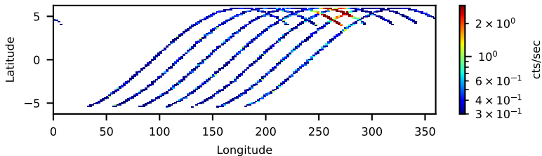
60160625002: 30 to 120 keV
