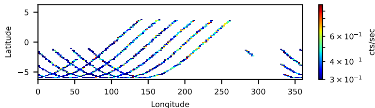
60160623002: 30 to 120 keV
