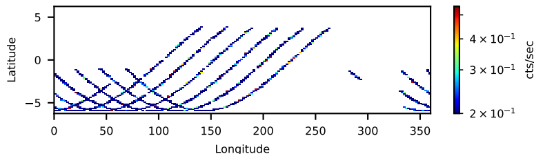
60160623002: 3 to 10 keV
