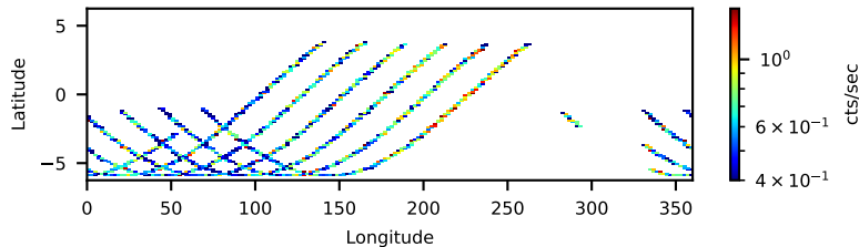
60160623002: 3 to 120 keV
