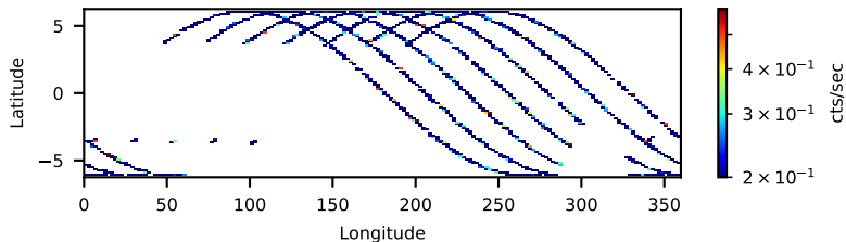
60160616002: 3 to 10 keV
