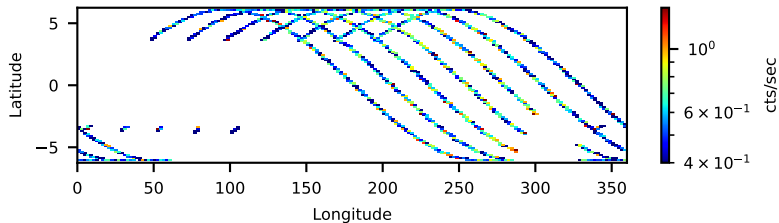
60160616002: 3 to 120 keV
