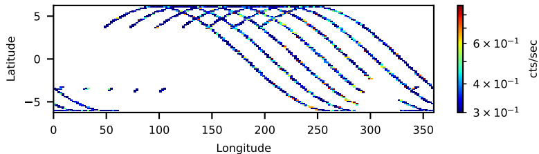
60160616002: 30 to 120 keV
