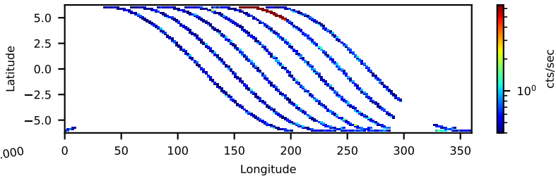
60160580002: 3 to 10 keV
