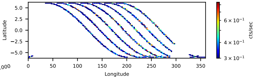
60160580002: 30 to 120 keV
