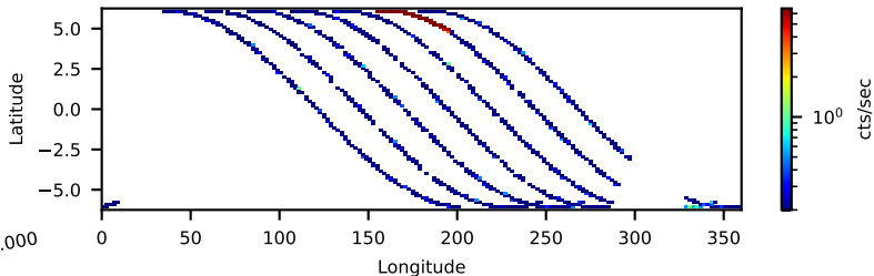
60160580002: 30 to 120 keV
