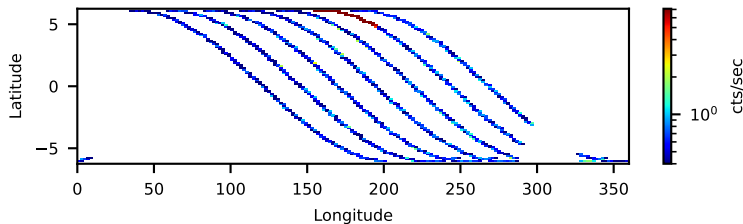
60160580002: 3 to 120 keV
