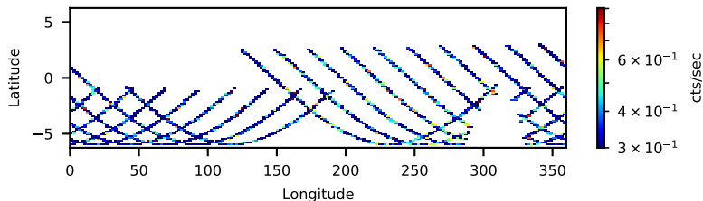
60160512002: 30 to 120 keV
