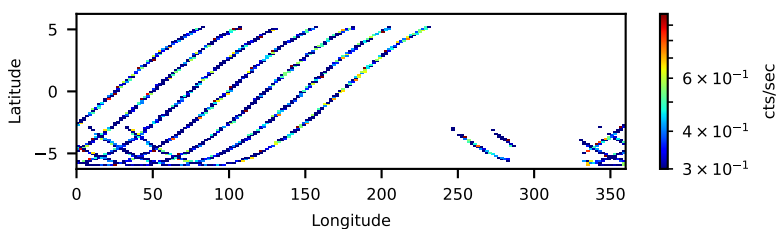
60160507002: 30 to 120 keV
