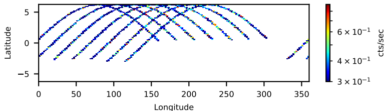
60160486002: 30 to 120 keV
