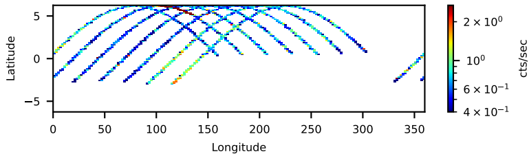
60160486002: 3 to 120 keV
