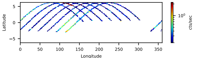
60160486002: 3 to 10 keV
