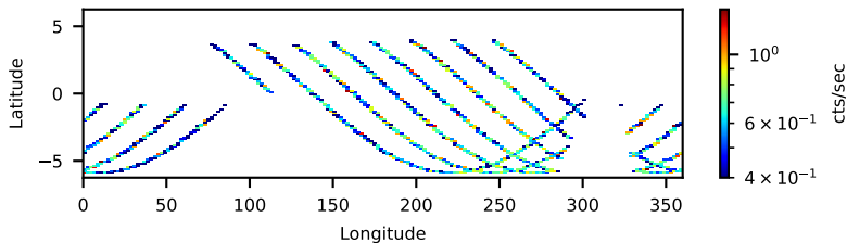
60160466002: 3 to 120 keV
