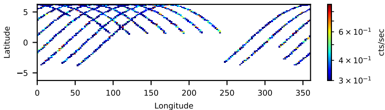
60160431002: 3 to 10 keV
