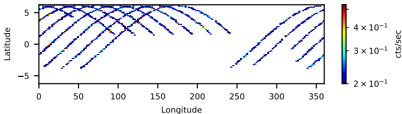
60160431002: 30 to 120 keV
