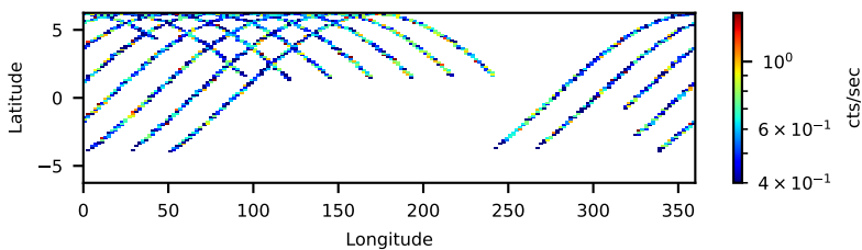
60160431002: 3 to 120 keV
