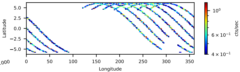
60160412002: 3 to 10 keV
