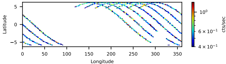
60160412002: 3 to 120 keV
