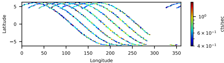
60160365002: 3 to 120 keV
