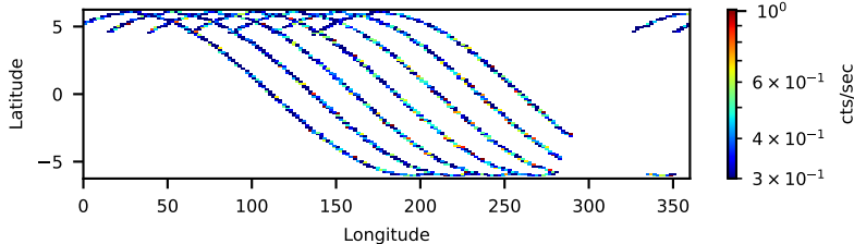
60160365002: 30 to 120 keV
