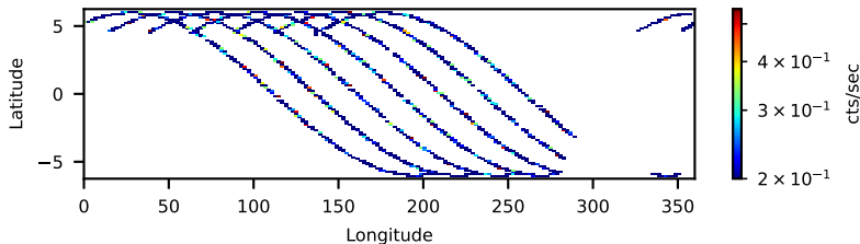
60160365002: 3 to 10 keV
