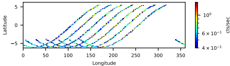
60160357002: 3 to 120 keV
