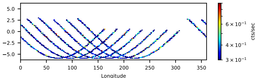
60160345002: 30 to 120 keV
