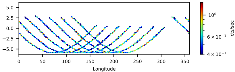
60160345002: 3 to 10 keV
