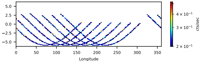
60160345002: 30 to 120 keV
